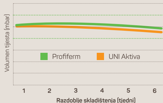
Volumen tijesta UNIFERM pekarskog kvasca
